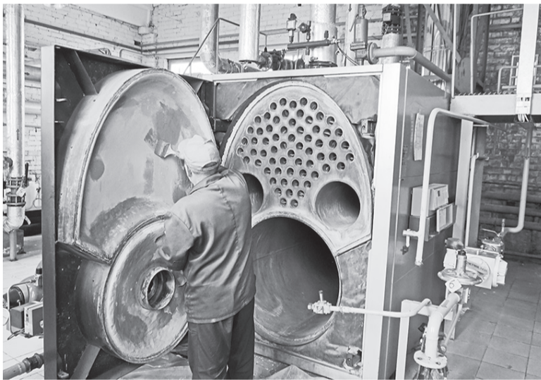
Подготовка фронтальной крышки котла
